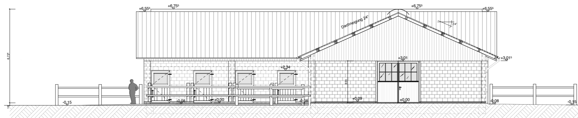
südansicht
